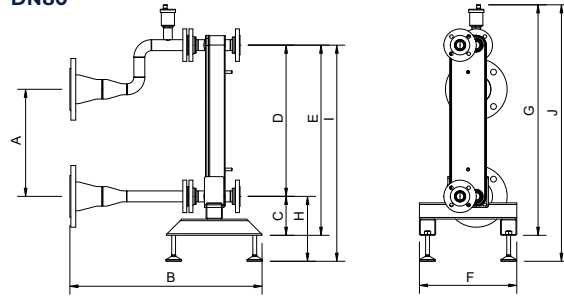
DN80
