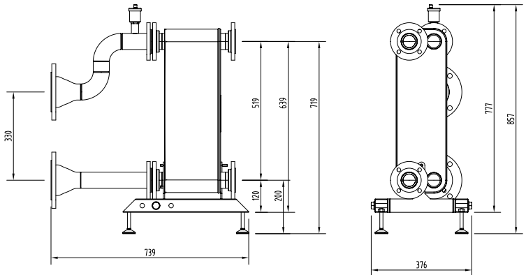
222226 DN80
