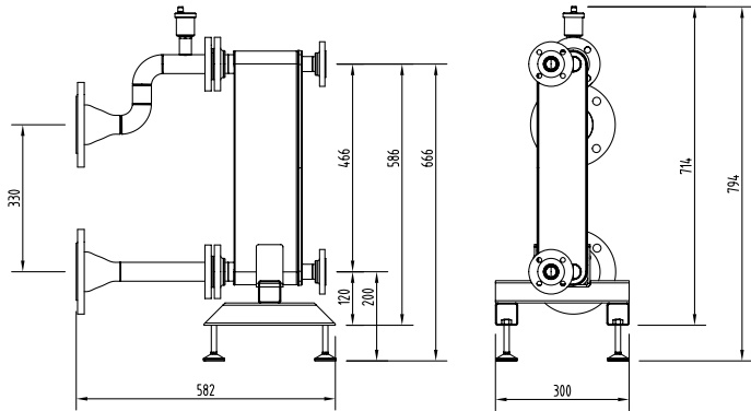
222994 DN65
