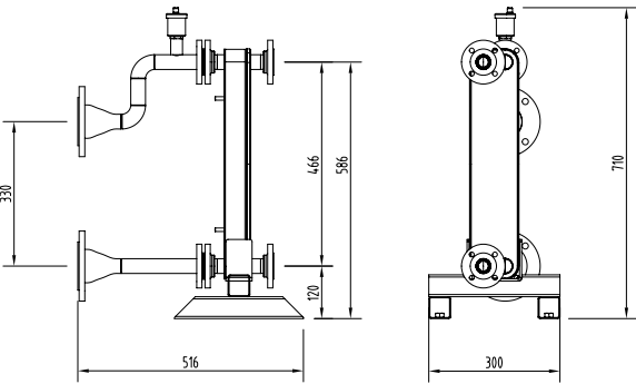
222993 DN65
