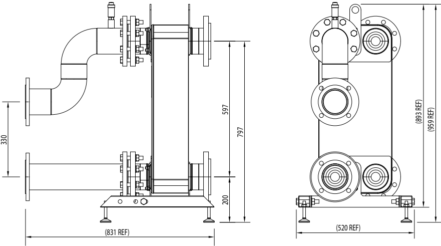
242216 DN100
