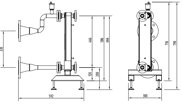
222220 DN80
