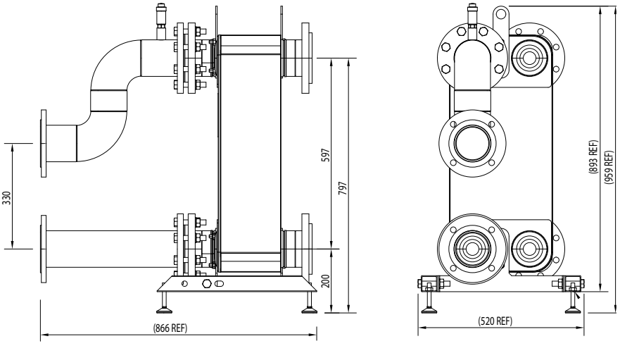
242217 DN100
