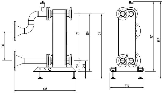
222995 DN100
