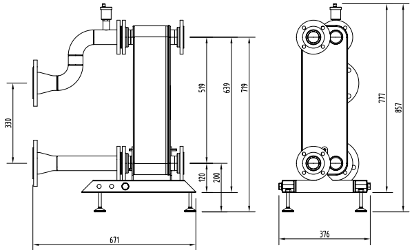
222225 DN80
