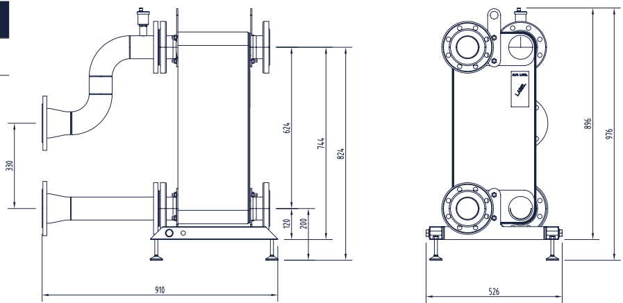
242217 DN150
