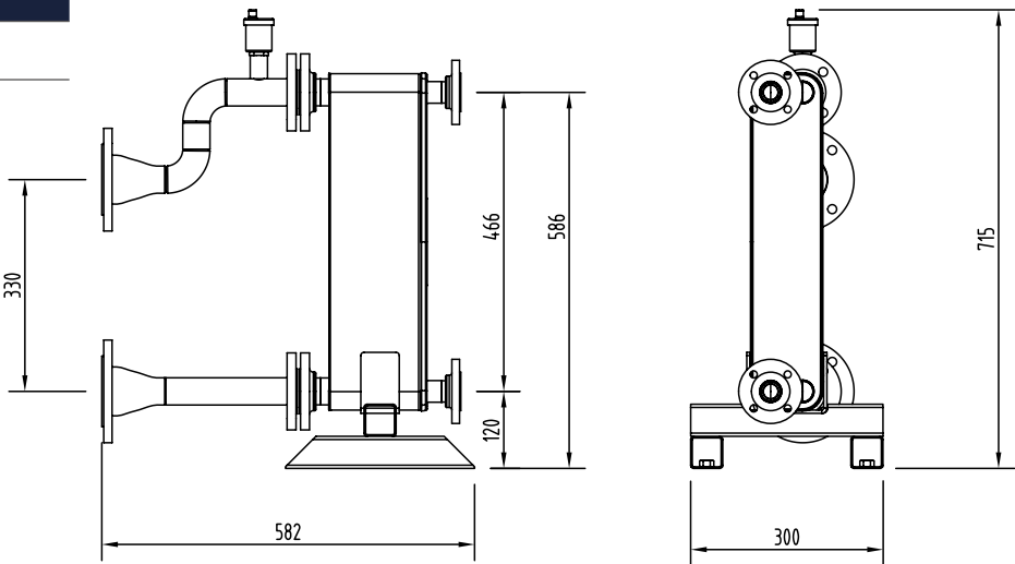
222222 DN80
