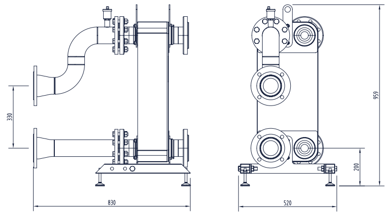
242216 DN100
