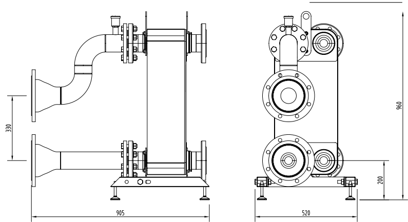
242219 DN150
