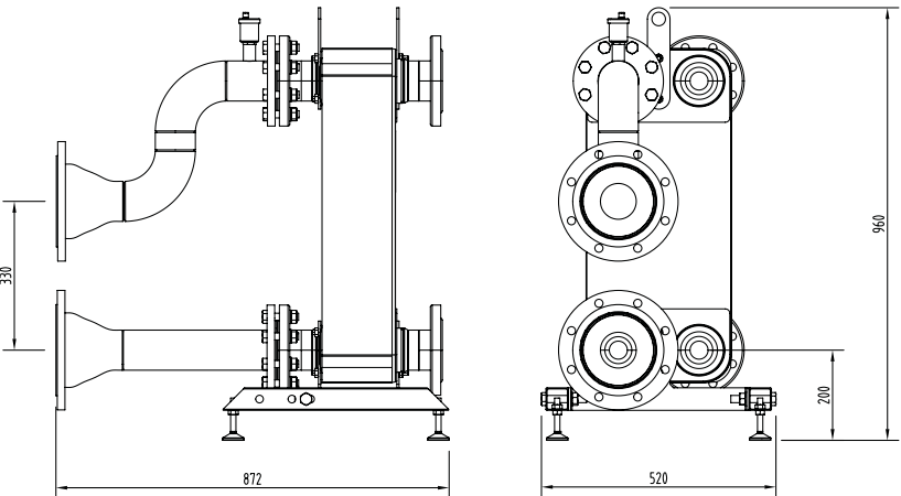
242218 DN150
