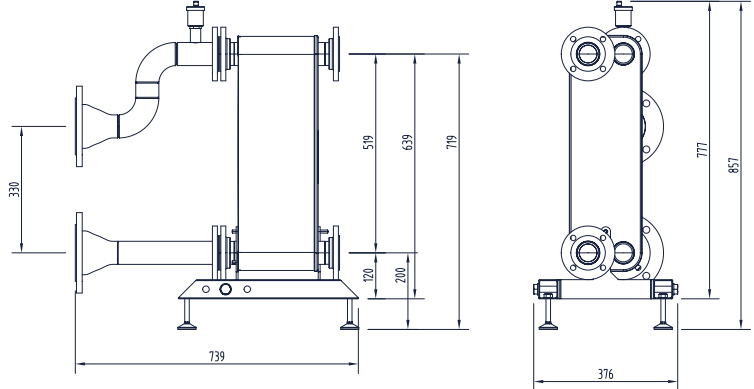
222226 DN80
