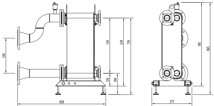
222227 DN100
