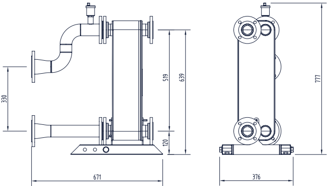
222223 DN65
