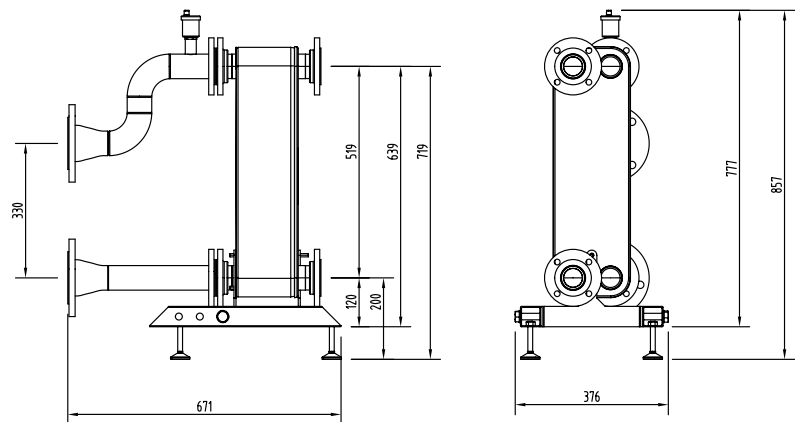
222225 DN80
