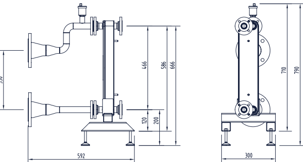
222220 DN80
