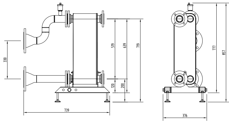
222226 DN80
